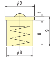
ボールカップ8.0 球帽 8.0
