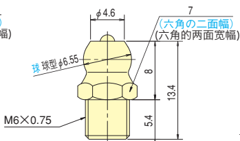
A M6 細目 细牙 (M6x0.75)
