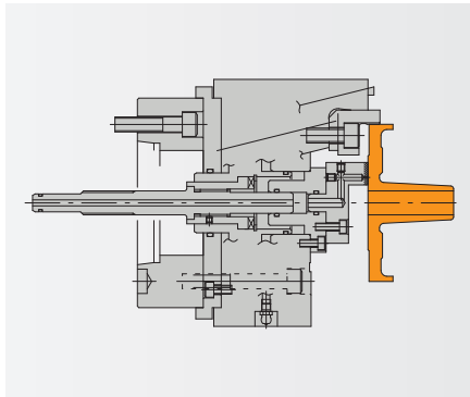
● シャフト
