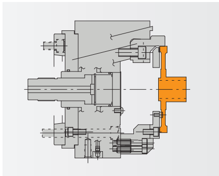
● ギア
