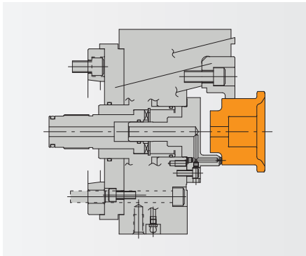
● ハブ
