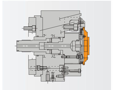
● ケース
