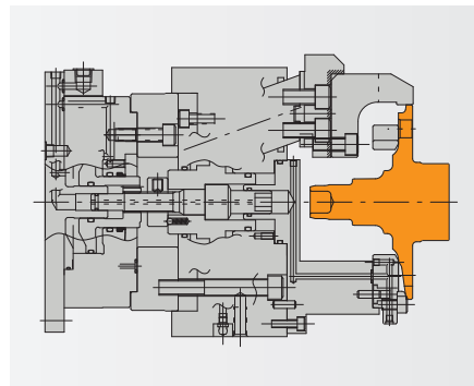
●ハブ
