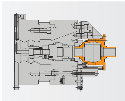
●ケース
