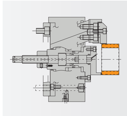
●ハブ
