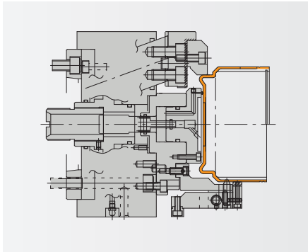
●プーリー
