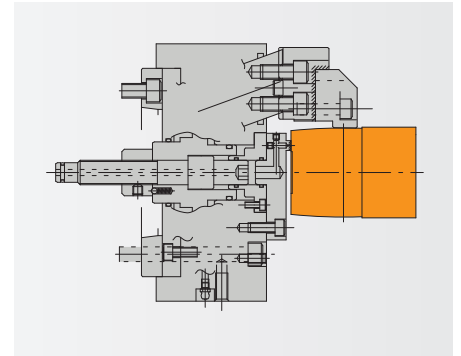
●ハブ
