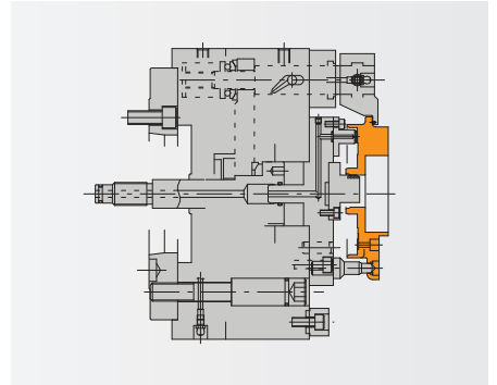
● ボディ
