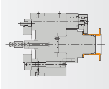
● ハブ
