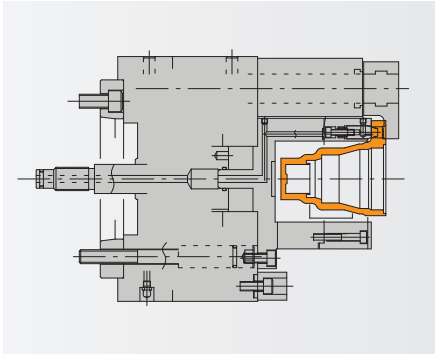
● ボディ
