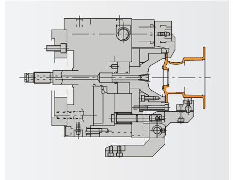
● ハブ
