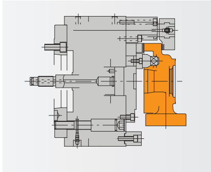
● ケース
