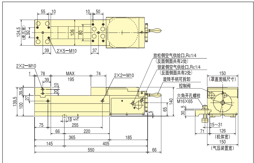
■ 尺寸图
